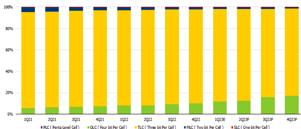
圖七 全球 Nand Flash 產量依產品架構分析
