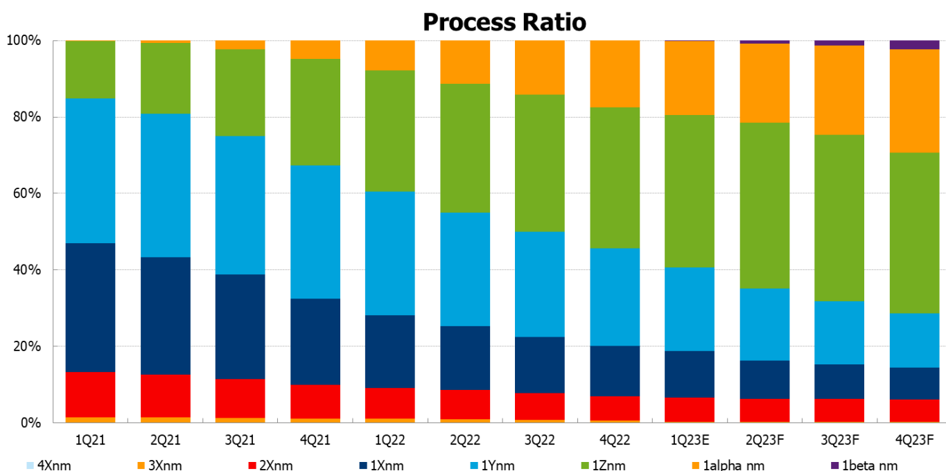
圖五 DRAM 製程演進
